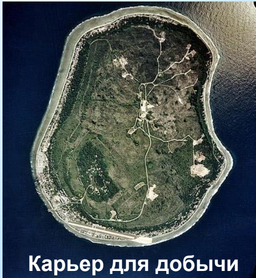
фосфориты
